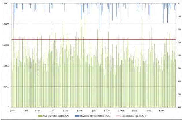
Figure 40 : DBO5 : flux journaliers entrants et pluviométrie - 2011
