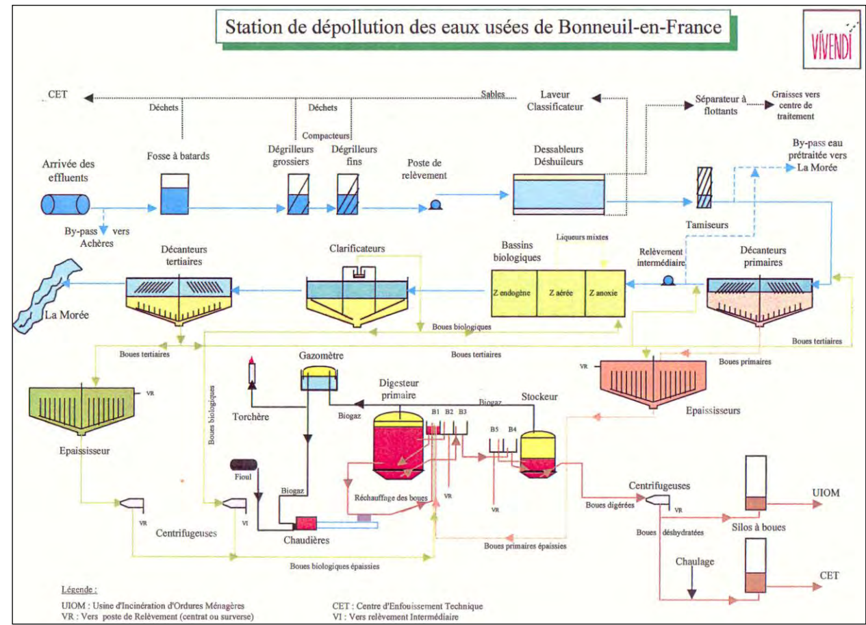
Figure 37 : synoptique de la station d'épuration du SIAH (source : OTV)
