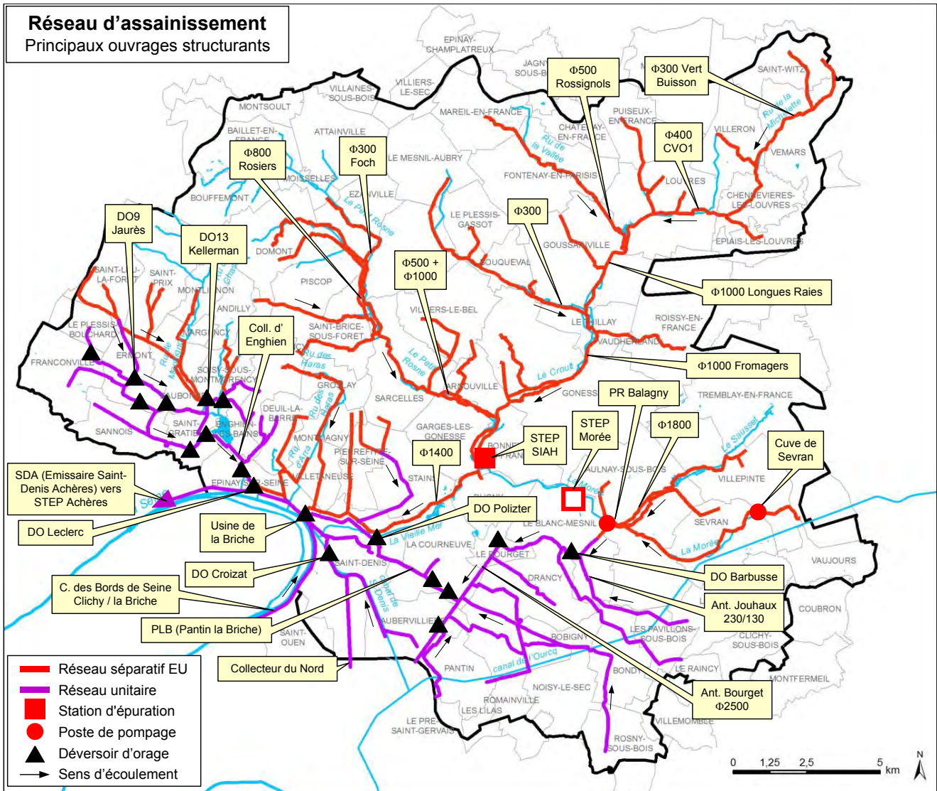
Figure 28 : Principaux ouvrages d'assainissement du territoire du SAGE
