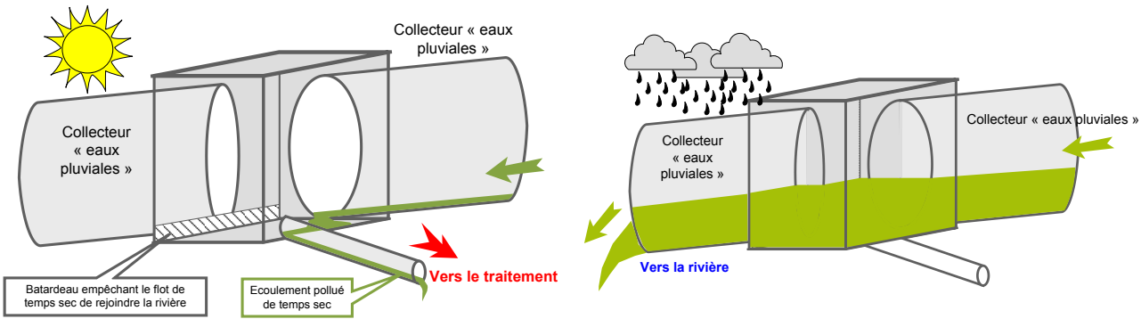
Figure 19 : Schéma simplifié d'une prise de temps sec sur collecteur pluvial
