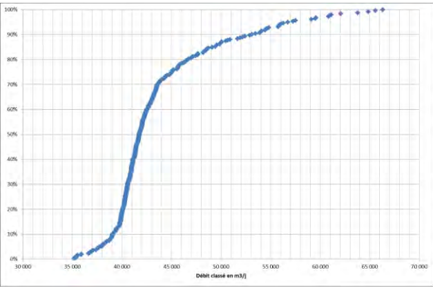
Figure 39 : débits journaliers entrants classés
