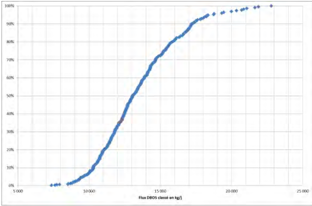
Figure 41 : DBO5 : flux journaliers entrants classés - 2011
